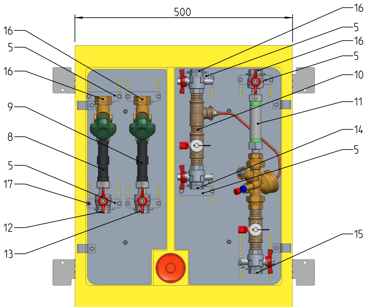
Ansicht ohne Tür
