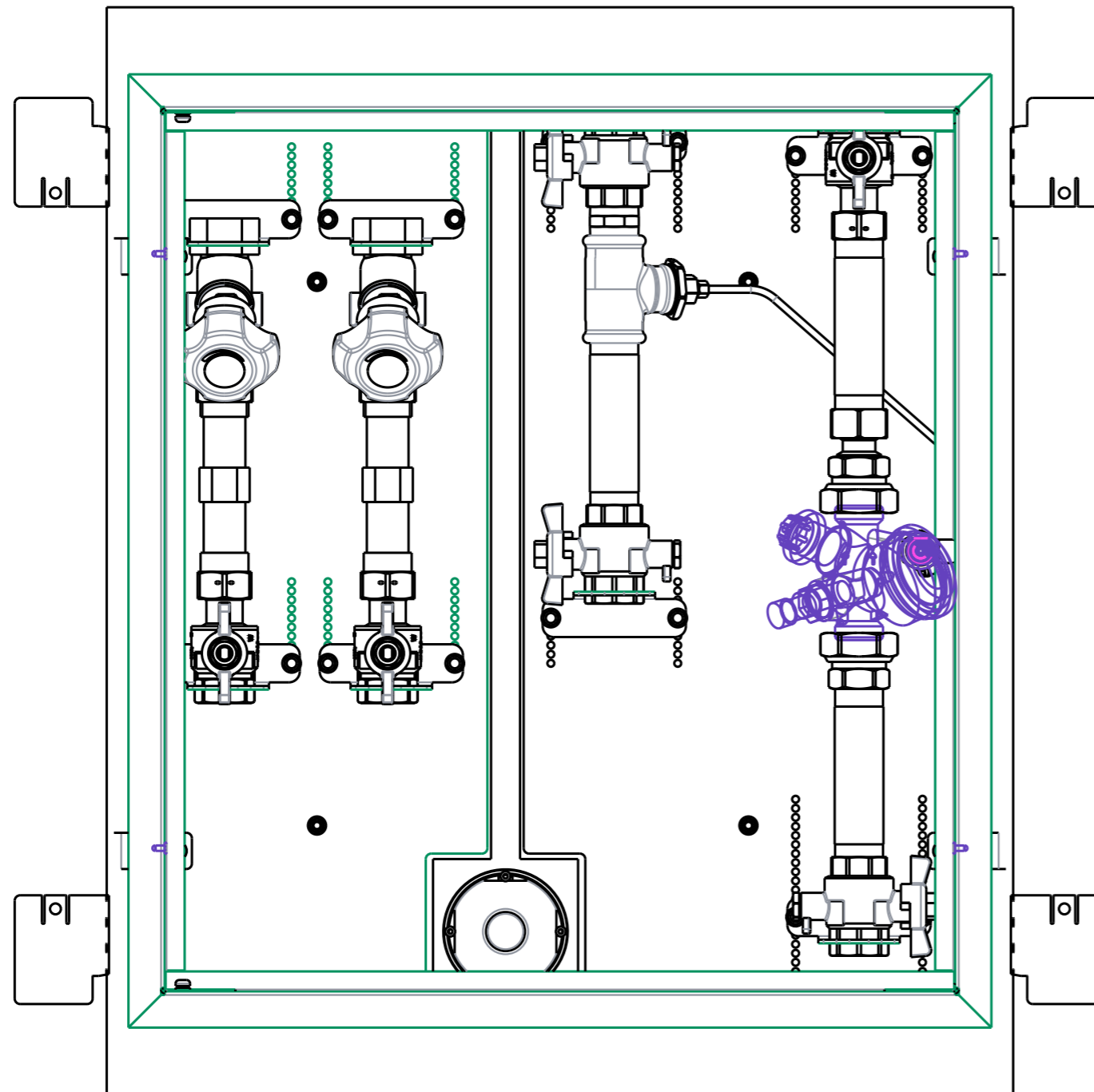
Ansicht ohne Türblatt
