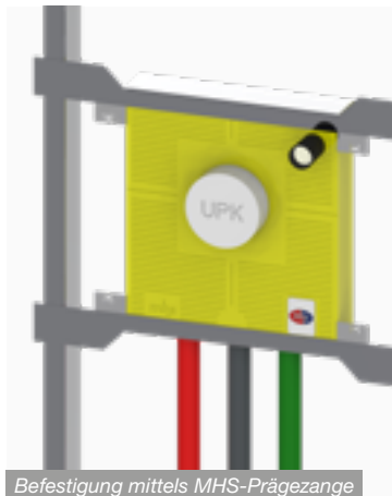
Befestigung mittels MHS-Prägezange
