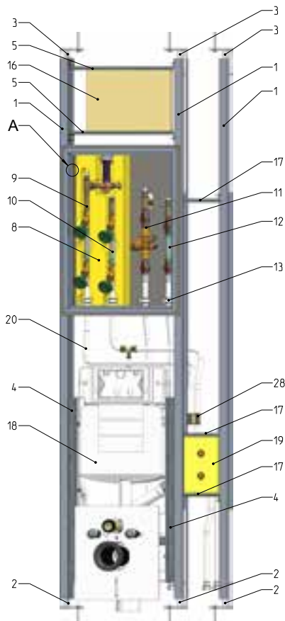
Ansicht ohne Türblatt/Box-Deckel
