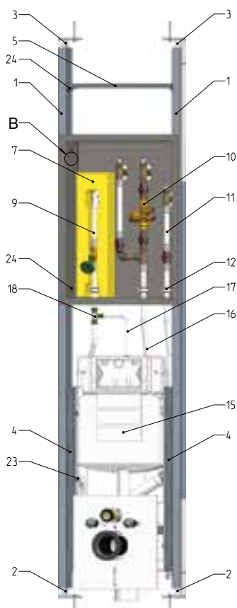
Ansicht ohne Türblatt/Box-Deckel
