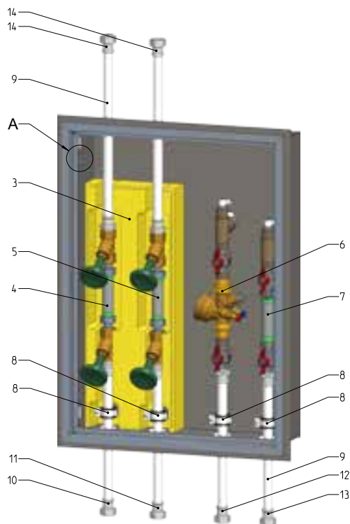
Ansicht ohne Türblatt/Boxdeckel
